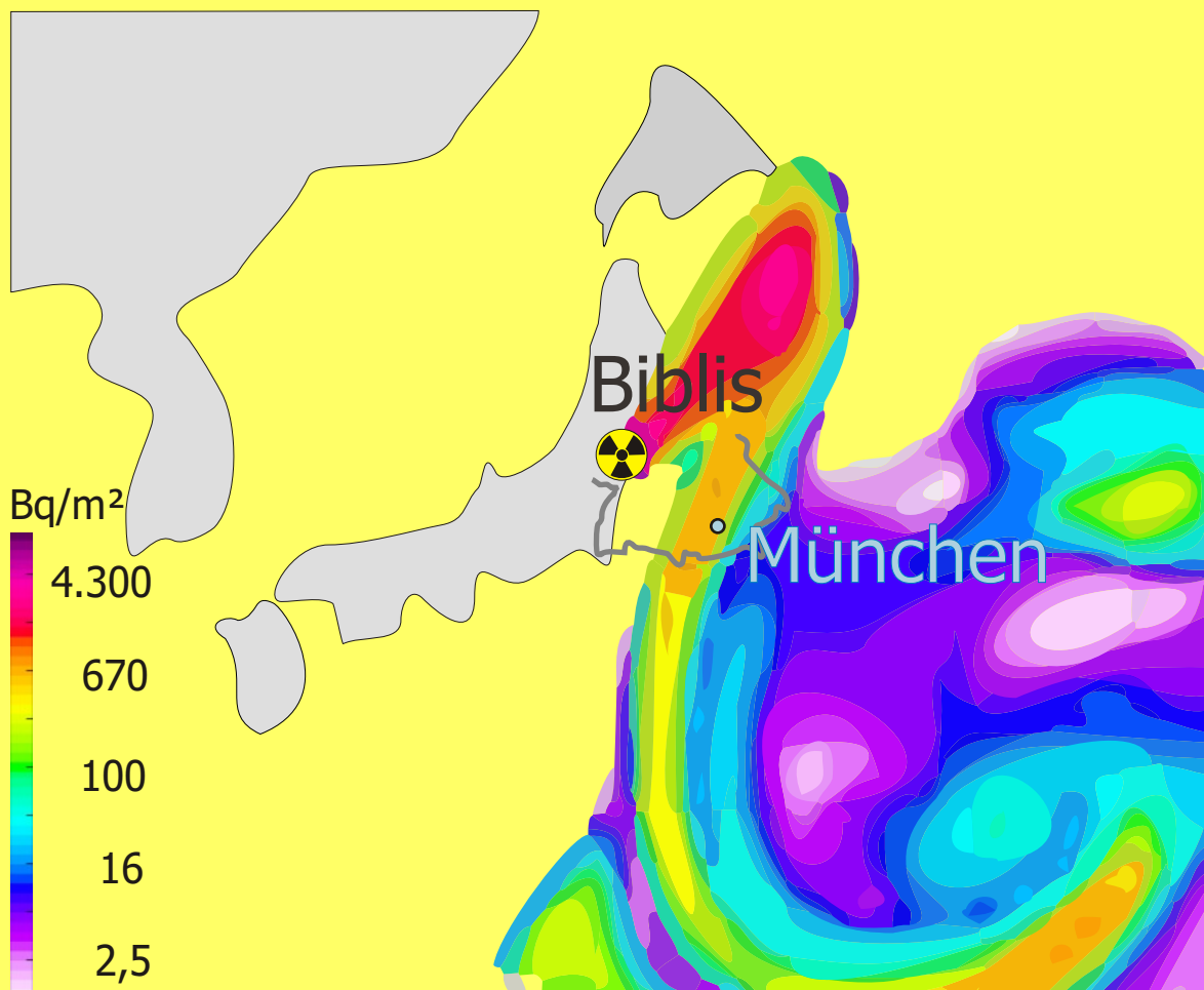
Zeitschrittansicht der Fukushima-Wolke (Jod 131) nach NILU-ATMOS Ausbreitungssimulation
