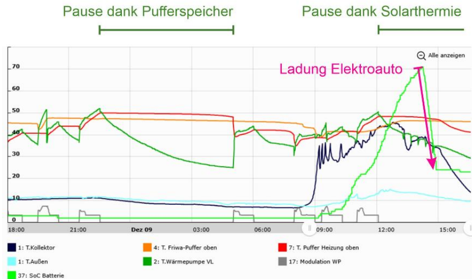
Wärmepumpenheizung mit 2 x 500 Liter Puffer und 5 m 2 Sonnenkollektor
